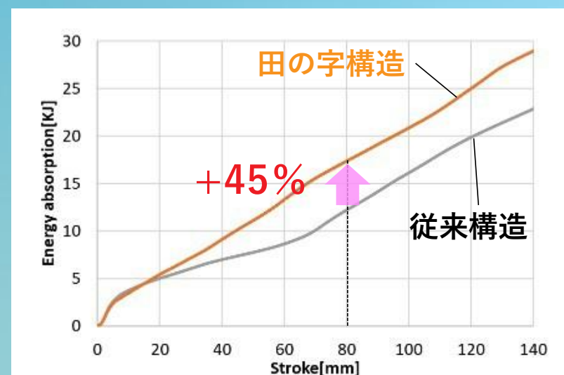
従来構造 軸圧潰性能 (重量同等)
