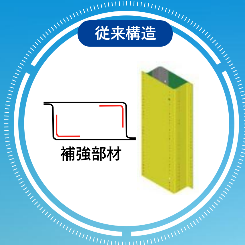
従来構造 軸圧潰性能 (重量同等)
