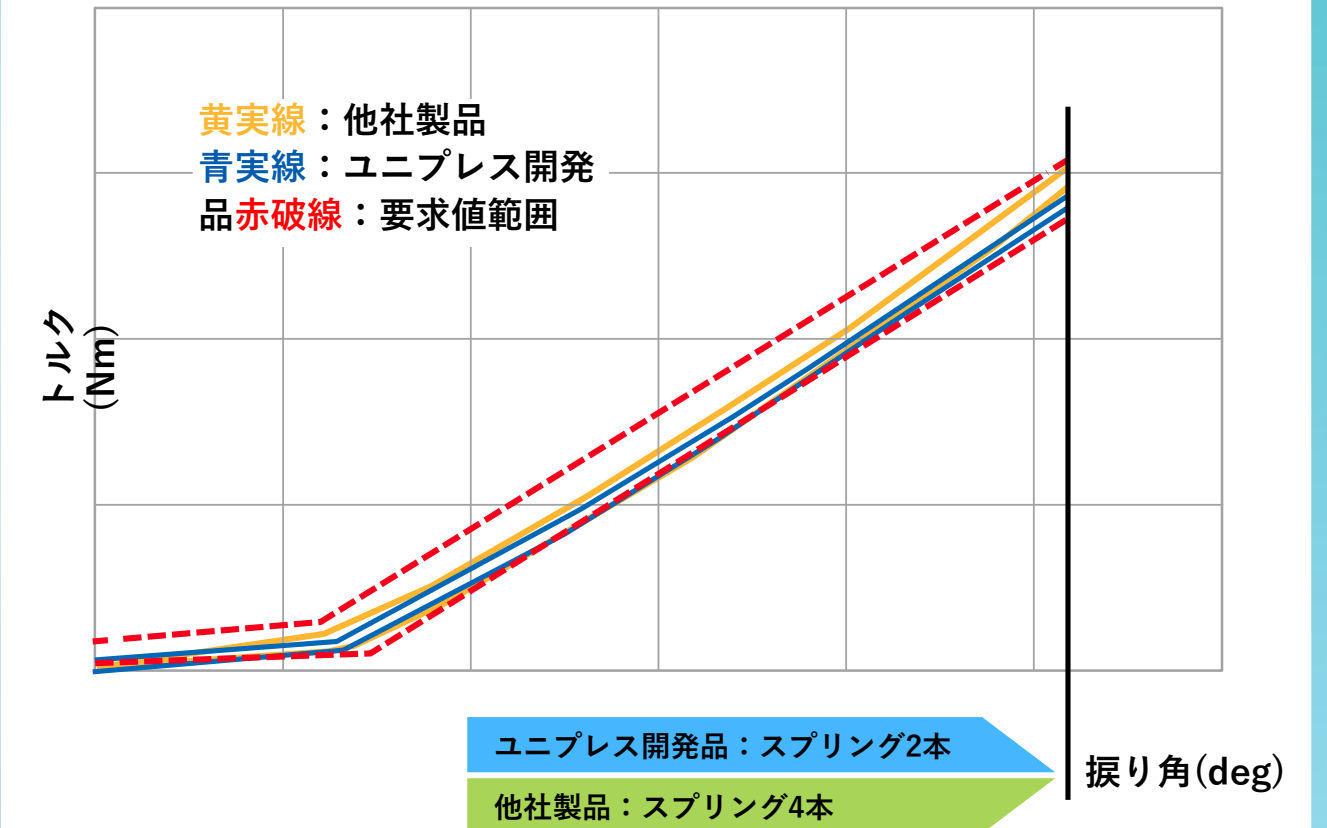
【ダンパ基本スプリング特性比較】
