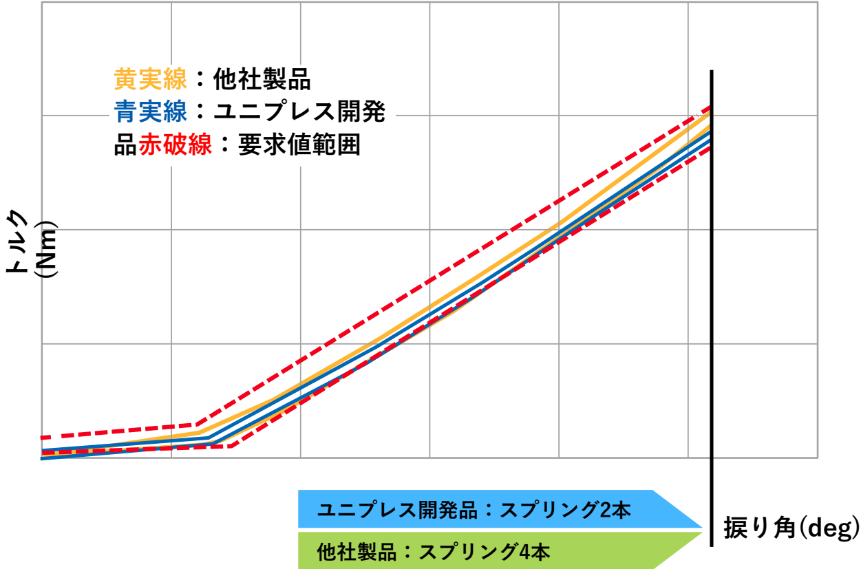
【ダンパ基本スプリング特性比較】
